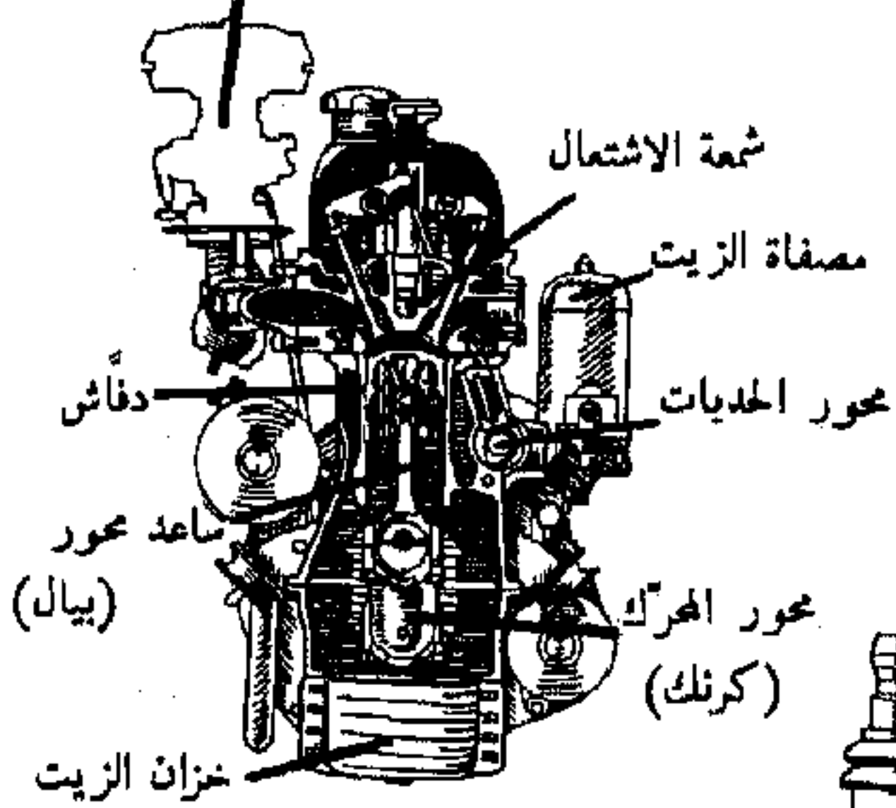
محرك : تصميم عمودي
